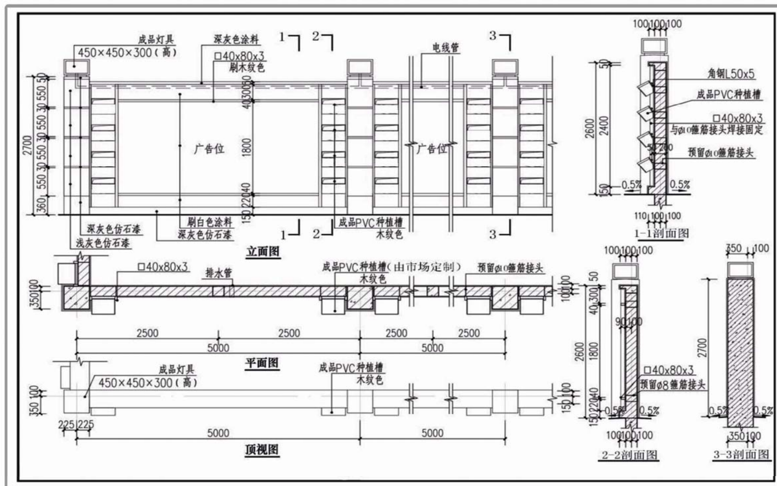
砖砌式围挡施工图一（造型部分）
